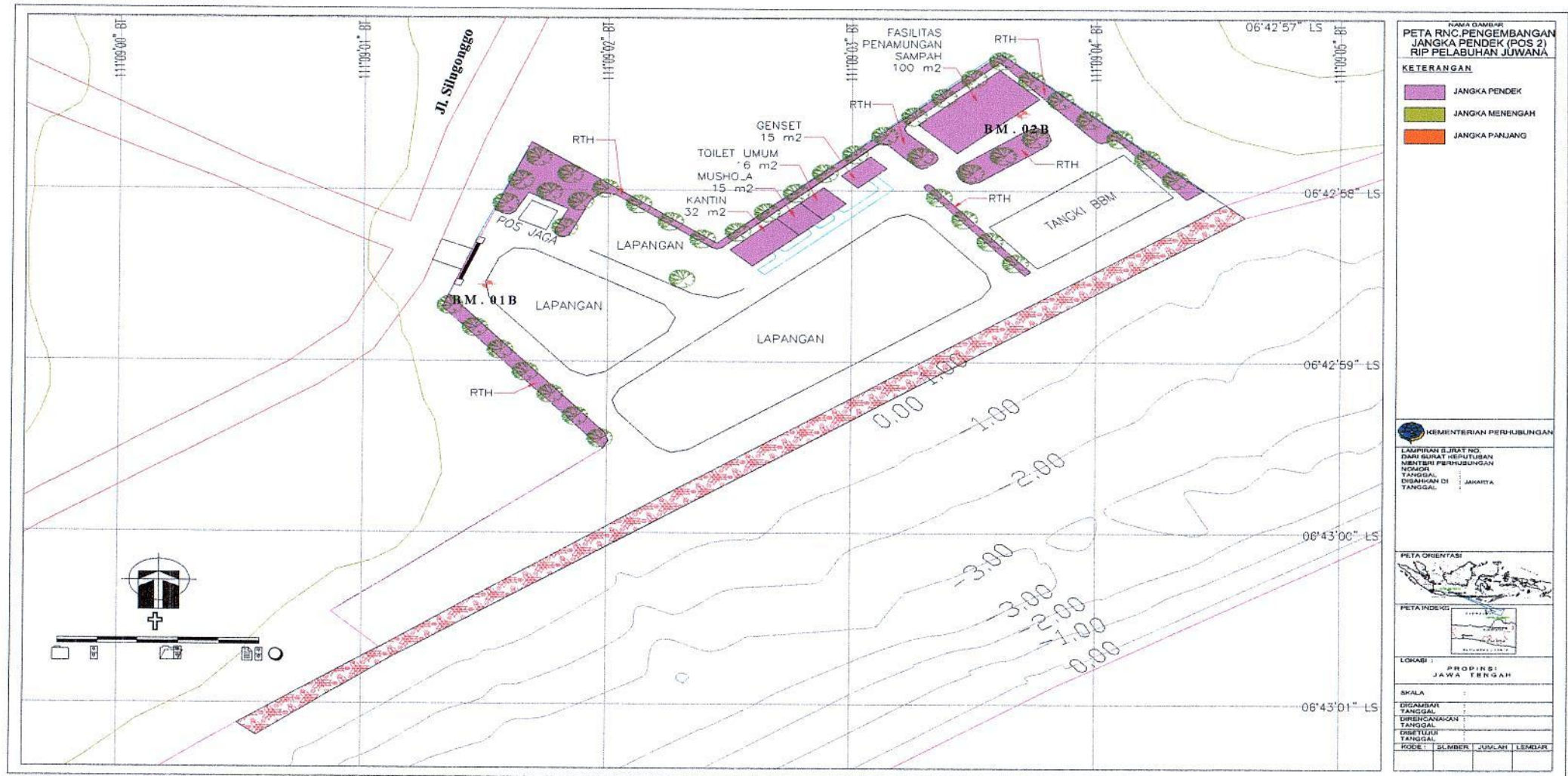
Gambar 31 Layout Pengembangan Pelabuhan Juwana Pos 2 Jangka Pendek Tahun 2017-2021
