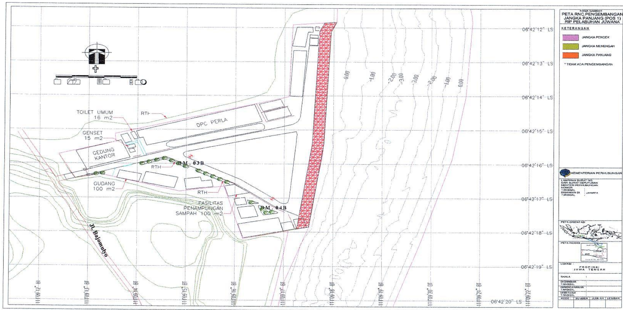
Gambar 30 Rencana Pengembangan Pelabuhan Juwana Pos 1 Jangka Panjang Tahun 2017-2036 (Tidak Ada Pengembangan)
