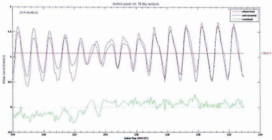
Gambar 12 Pengamatan Pasang Surut Air Laut Selama 15 Hari
