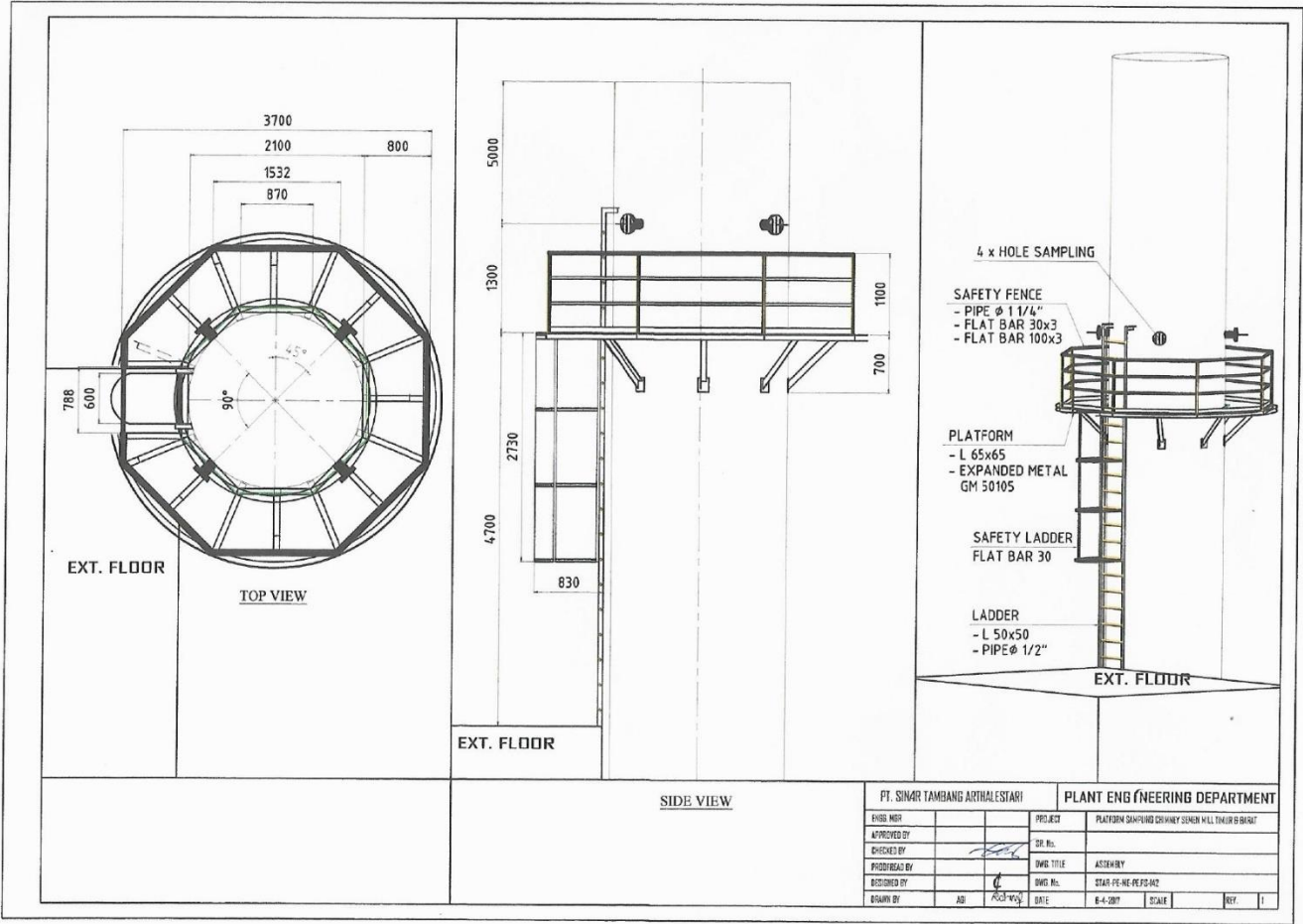
Gambar 53. Sarana dan Prasarana Pengambilan Sampel di Cerobong Cement Mill 1
