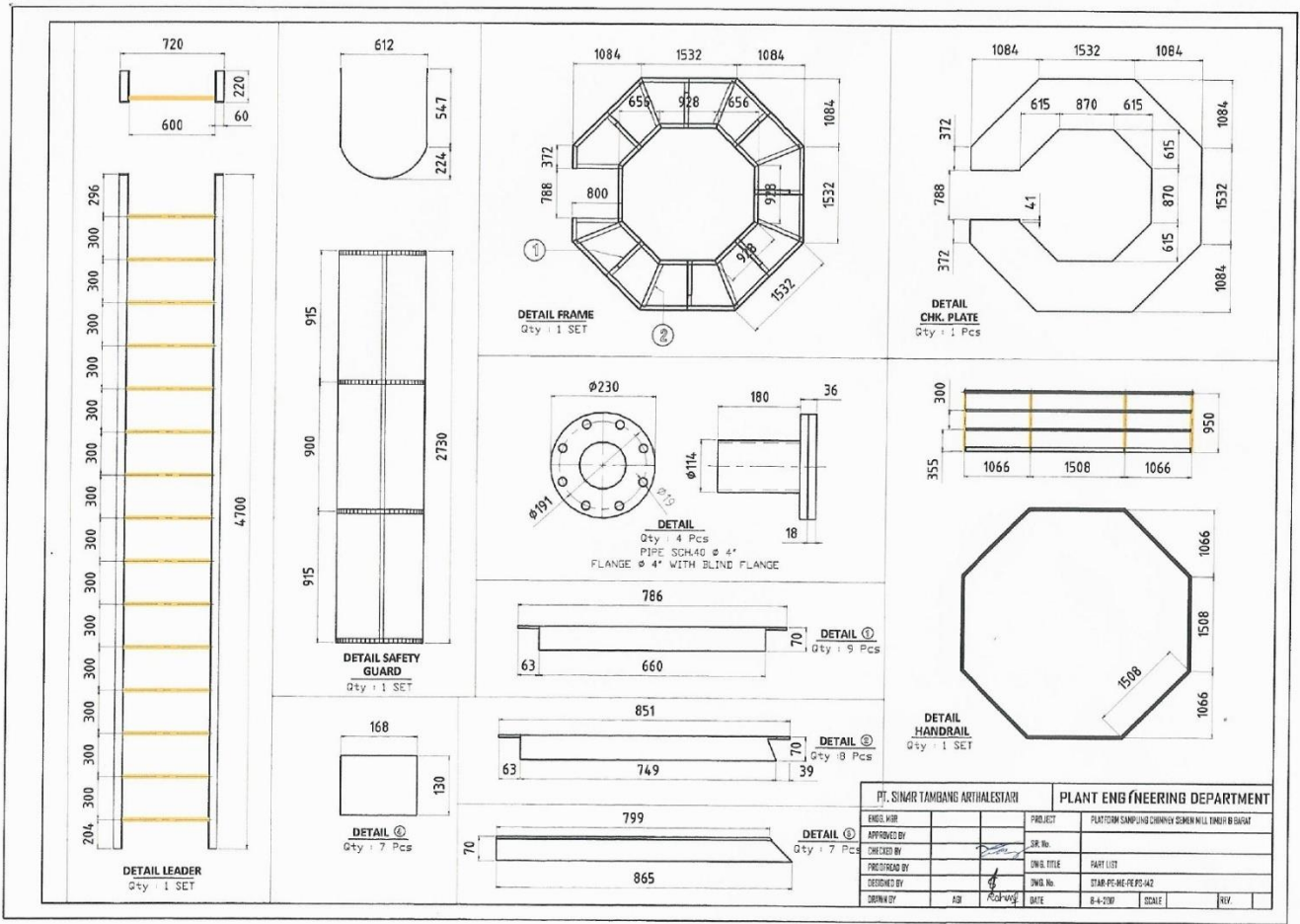
Gambar 57. Sarana dan Prasarana Pengambilan Sampel di Cerobong Cement Mill 2
