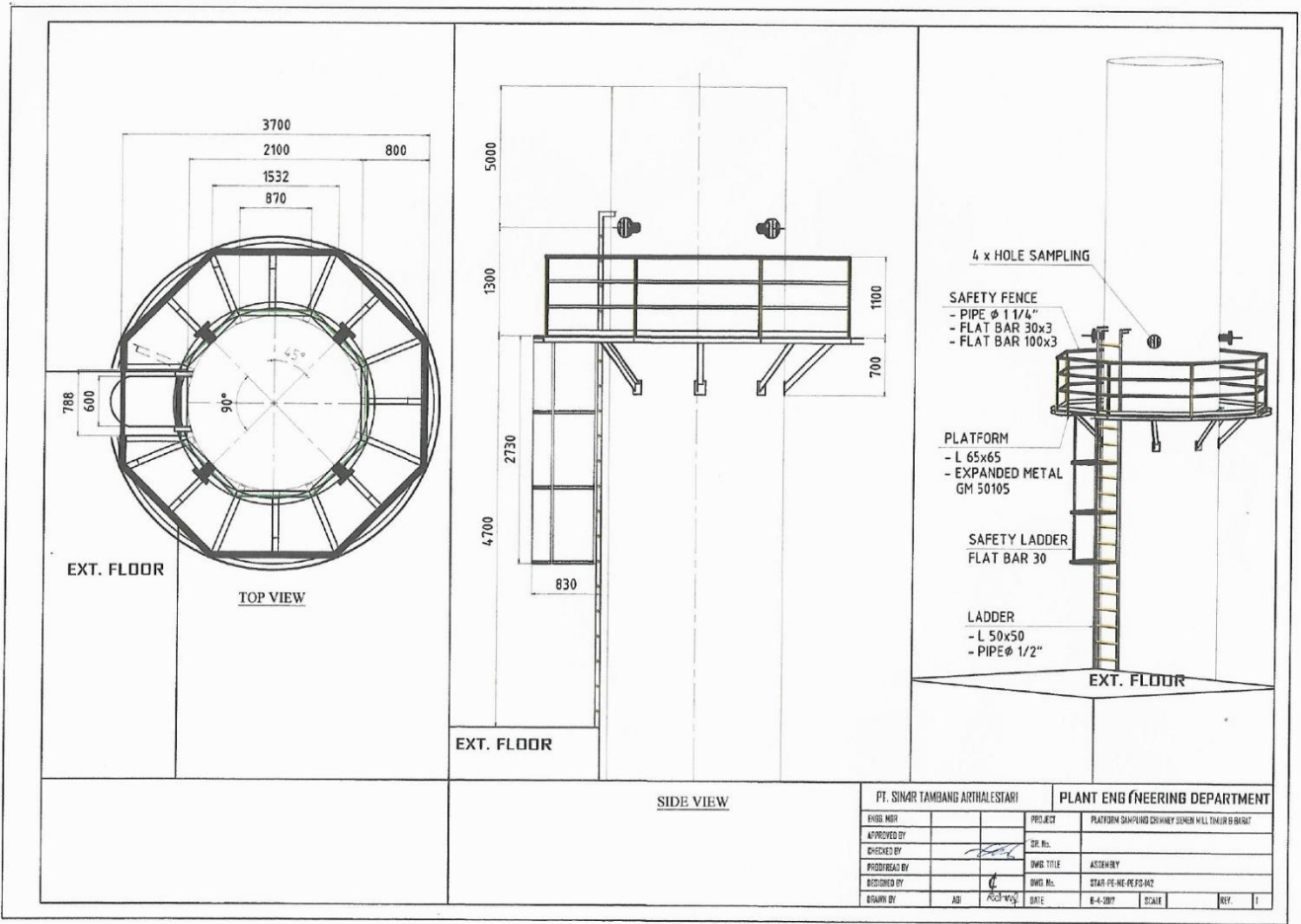
Gambar 56. Sarana dan Prasarana Pengambilan Sampel di Cerobong Cement Mill 2
