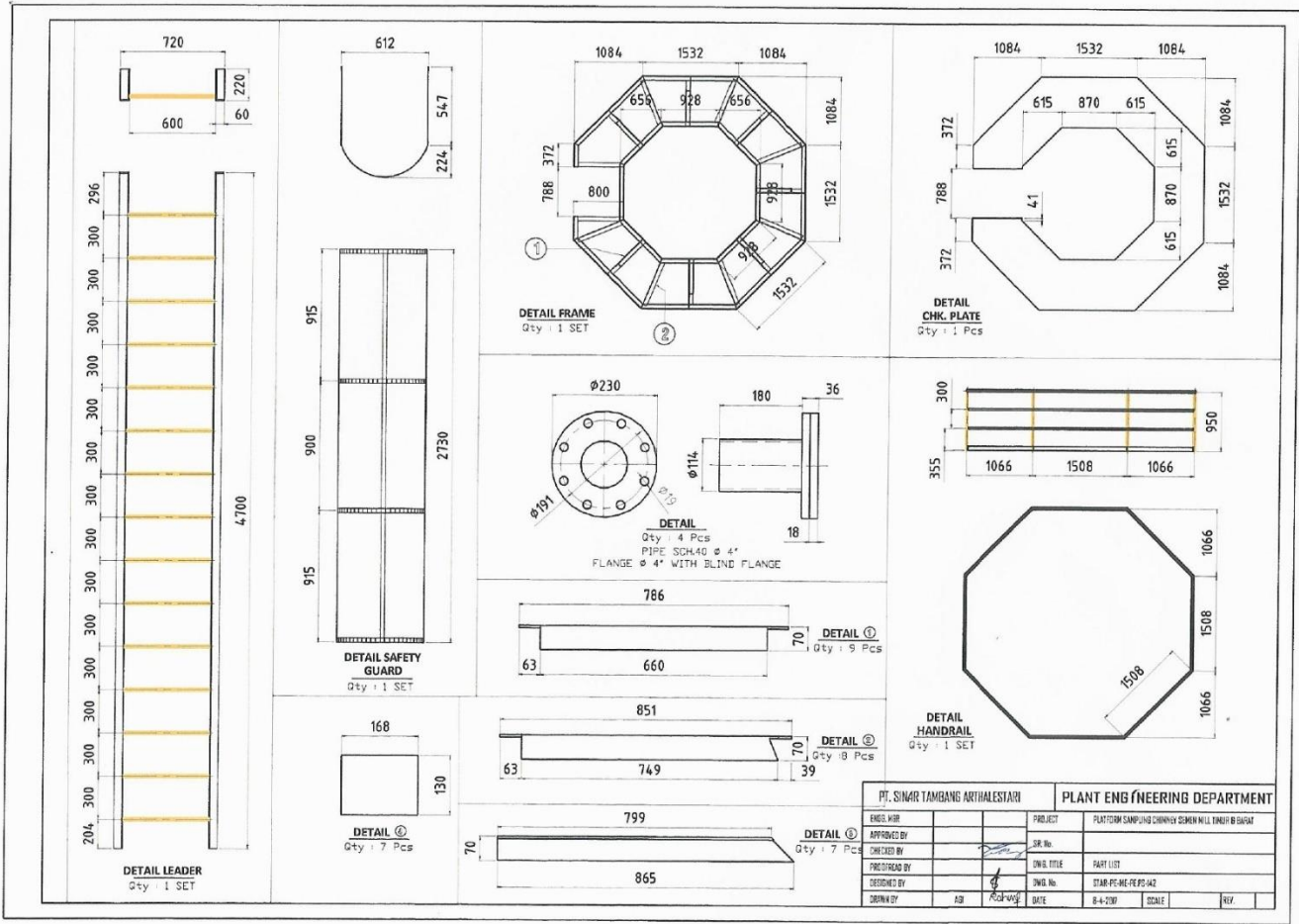
Gambar 54. Sarana dan Prasarana Pengambilan Sampel di Cerobong Cement Mill 1
