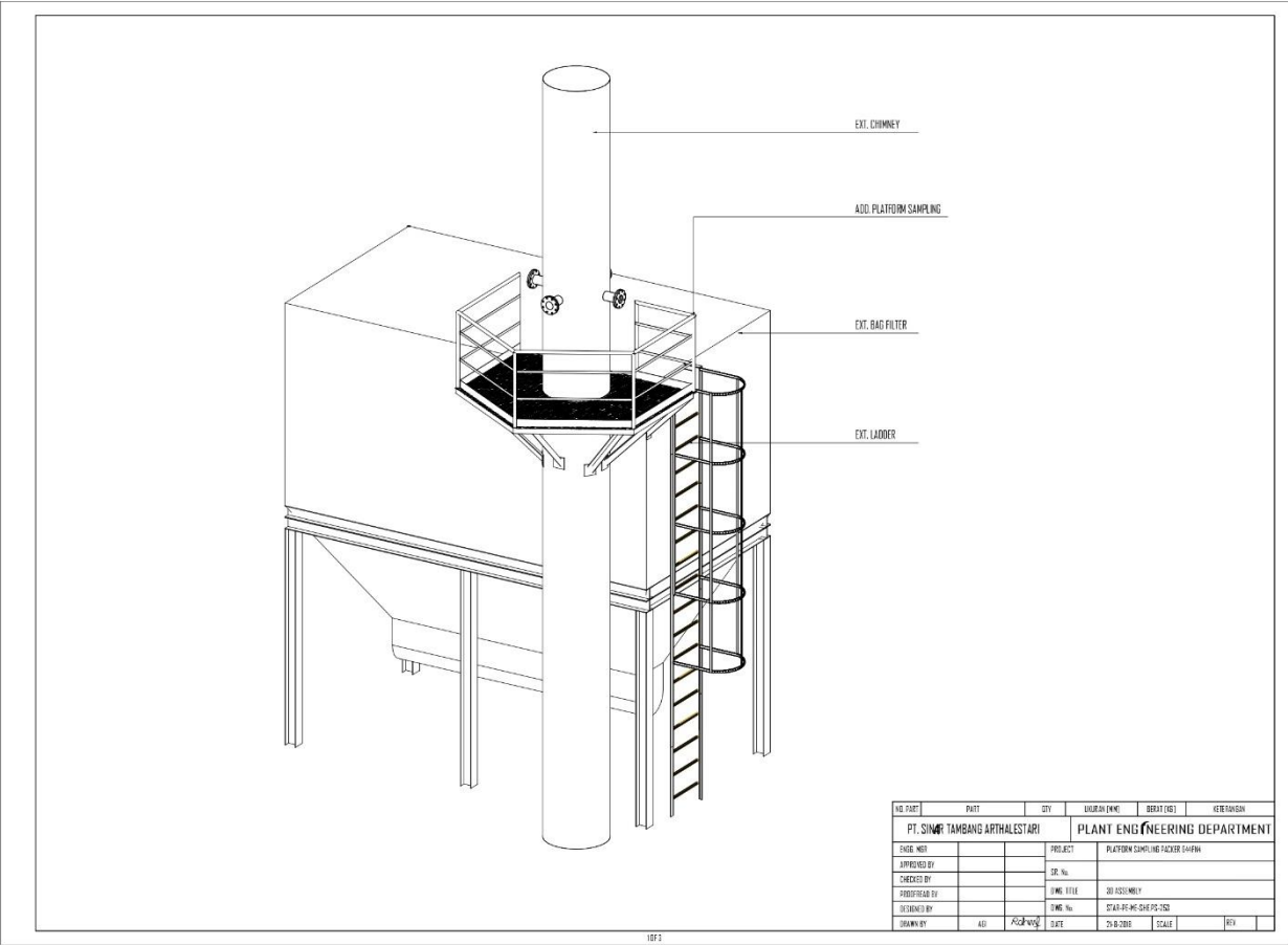
Gambar 68. Sarana dan Prasarana Pengambilan Sampel di Cerobong Cement Packer
